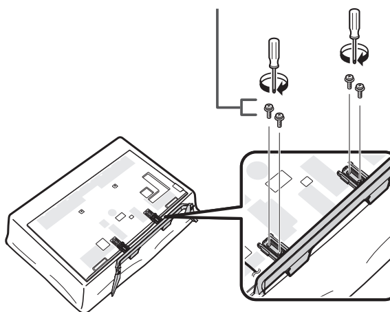
M5 schroeven
